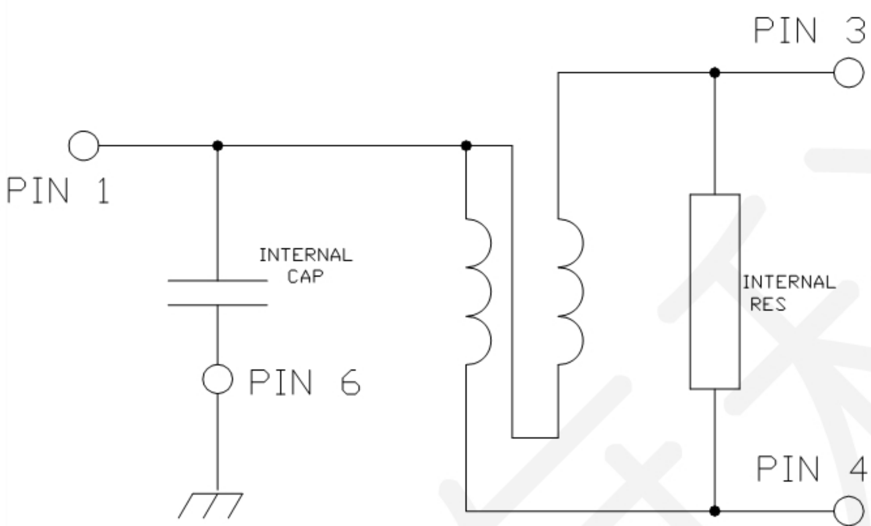
电气结构
