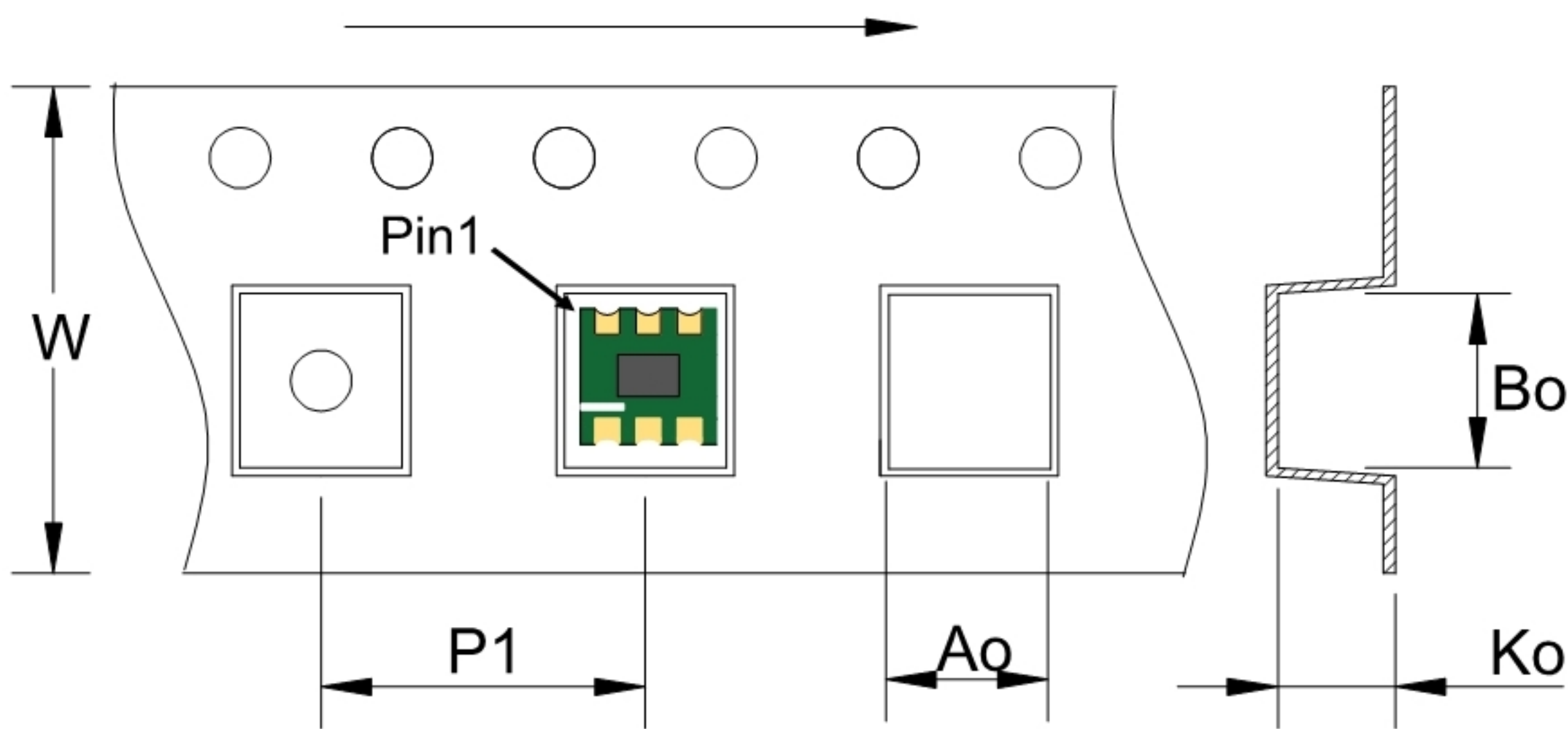
包装示意图
